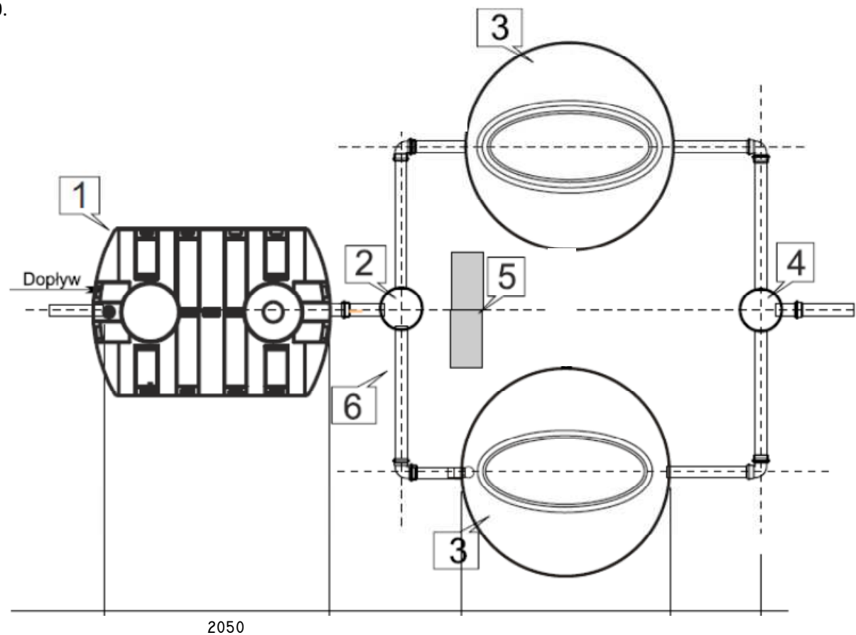
Rysunek 2 Oczyszczalnia ścieków Delfin Pensjonat 24 RLM
