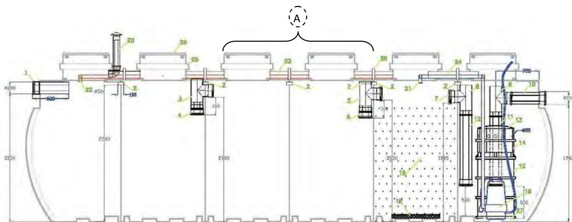
Rys.2. Osadnik wstępny – A
