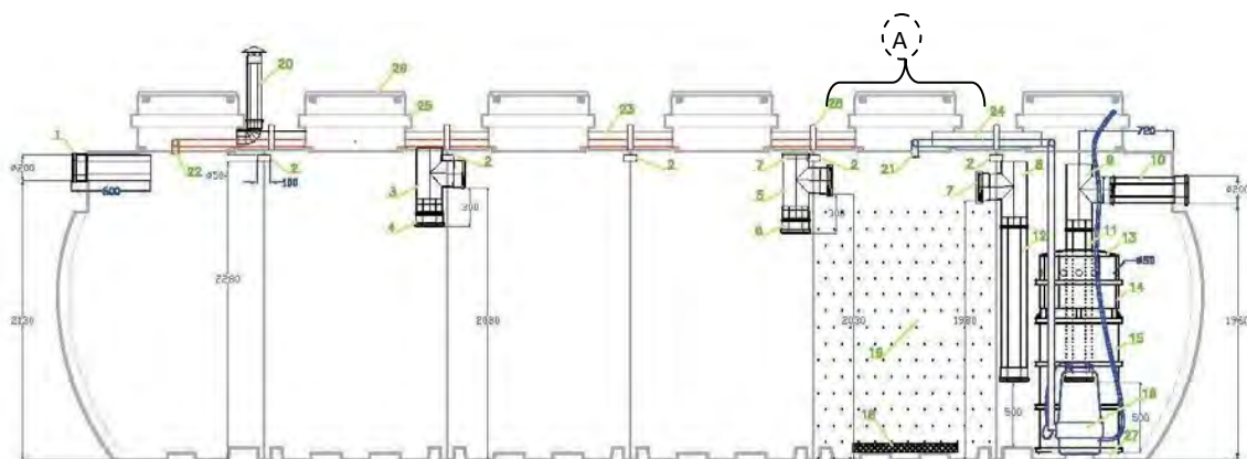
Rys.3. Komora napowietrzania – A
