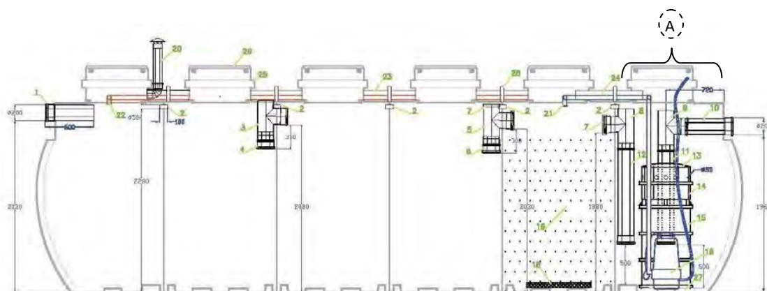
Rys.4. Osadnik wtórny – A
